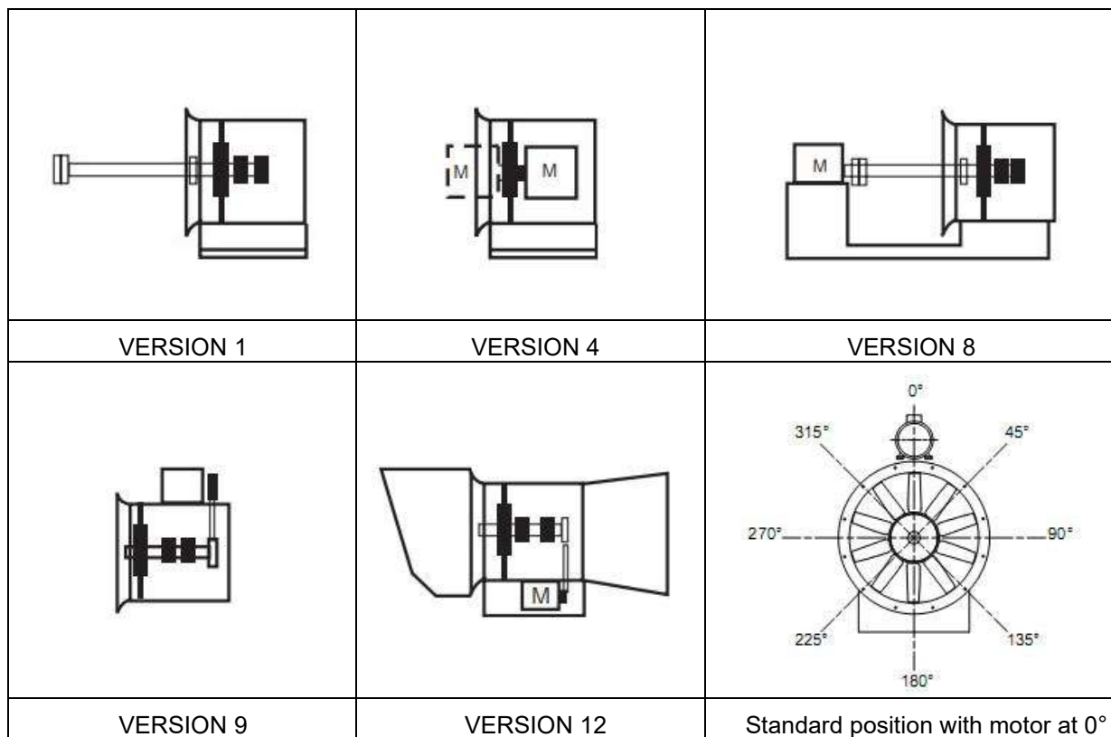
Fig. 2-1 Axial fan versions
